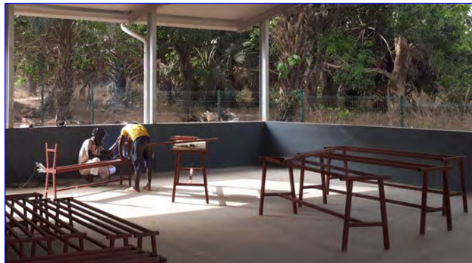
Si stanno costruendo i tavoli e le panche per la mensa scolastica. La struttura è in ferro mentre i piani sono in legno. Successivamente verranno costruite con la stessa tecnica le scaffalature per la cucina, per il deposito viveri e la biblioteca.
